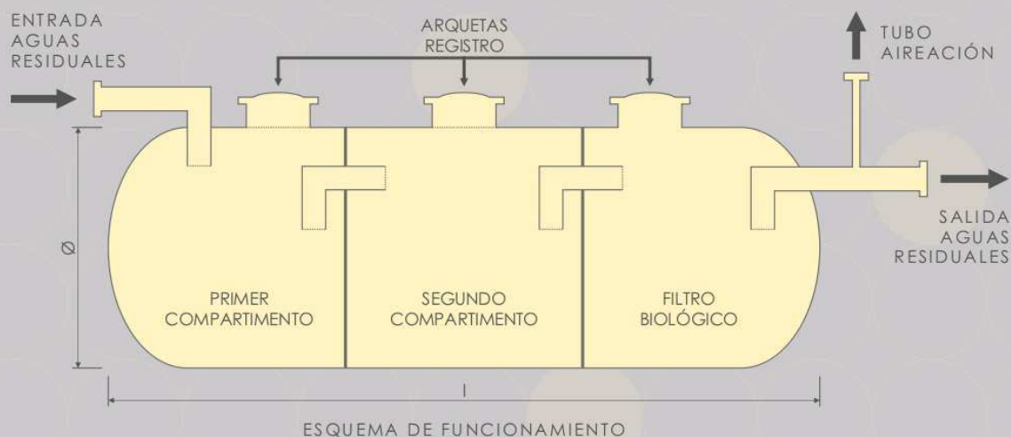
MODELO COMPACTO DECANTADOR - DIGESTOR FILTRO BIOLÓGICO
